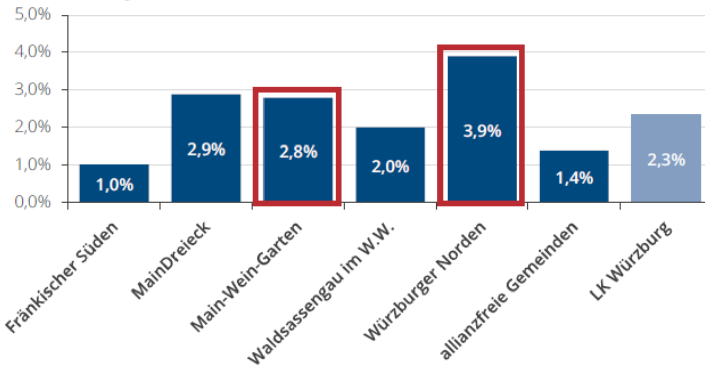
Entwicklung 2013-2019 in %
