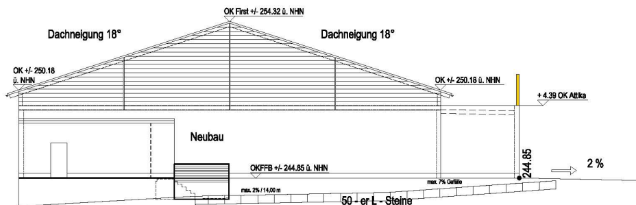
Nord - West Ansicht
